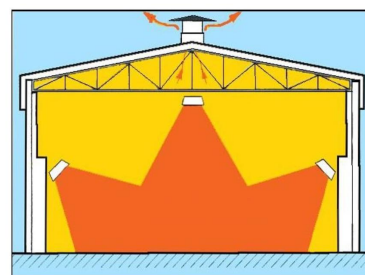
Zone chauffée par les radiants lumineux
